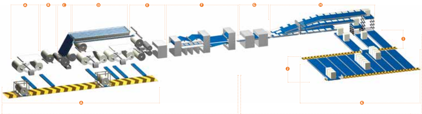
Ligne d'onduleuses
